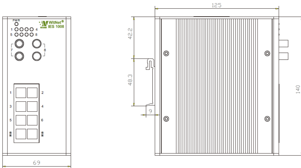
图 2-2 RugNet IES1008 结构尺寸图
